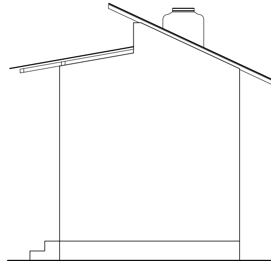
TAMPAK SAMPING KANAN Skala 1 : 75
