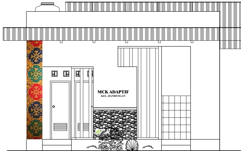
TAMPAK DEPAN Skala 1 : 75
