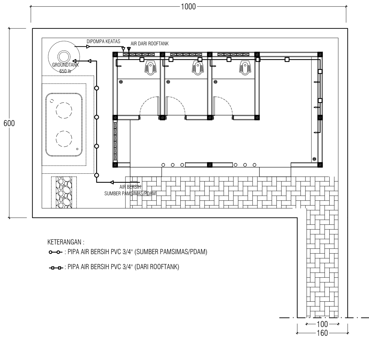
DENAH INSTALASI AIR BERSIH Skala 1 : 75
